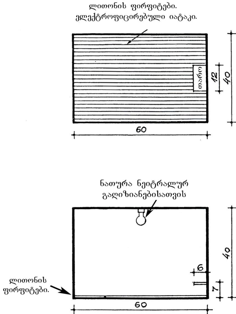
სურ. 3.1. აქტიური თავდაცვითი ქცევის გამოსამუშავებელი კაბინა
